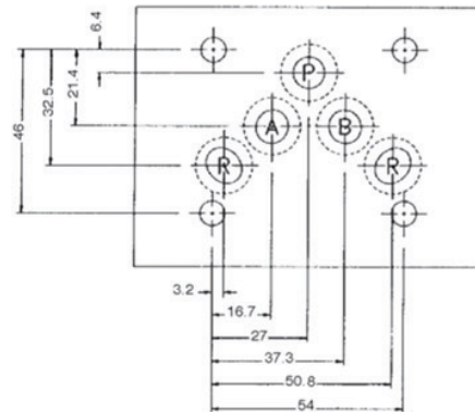
ISO 4401-AC-05-4-A - CETOP 05
