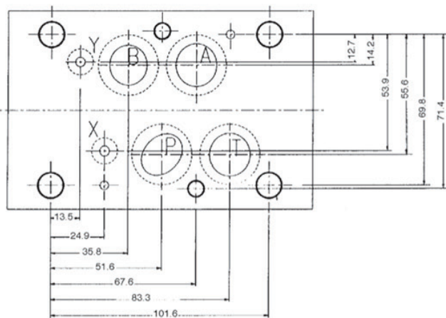
ISO 4401-AD-07-4-A - CETOP 07
